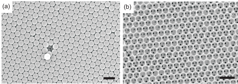
FIGUUR 4: Electronenmicroscopie afbeelding van een polystyreen opaal (de mal) en een lichtbolkristal. (a) Een kunstmatig opaal opgebouwd uit bolletjes met een doorsnede van 500 nanometer (schaalbalk is 500 nanometer). De bolletjes zijn mooi gerangschikt in een hexagonaal patroon. De structuur is drie-dimensionaal, zoals te zien aan het gat in het midden; hier mist een bolletje en zijn de beneden liggende bolletjes te zien. (b) Een lichtbolkristal van titaandioxide, de replica van een kunstmatig opaal. De diameter van de lichtbollen is 600 nanometer (de schaalbalk is 1500 nanometer) en zijn ook gerangschikt in hexagonaal patroon. De zwarte plekje noemen we “raampjes”; het zijn de plaatsen waar de bolletjes in de mal elkaar aanraakten en geen titaandioxide is afgezet.
